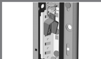
kotvení pružin
