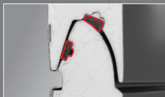
zdvojené robustnější těsnění mezi panely
